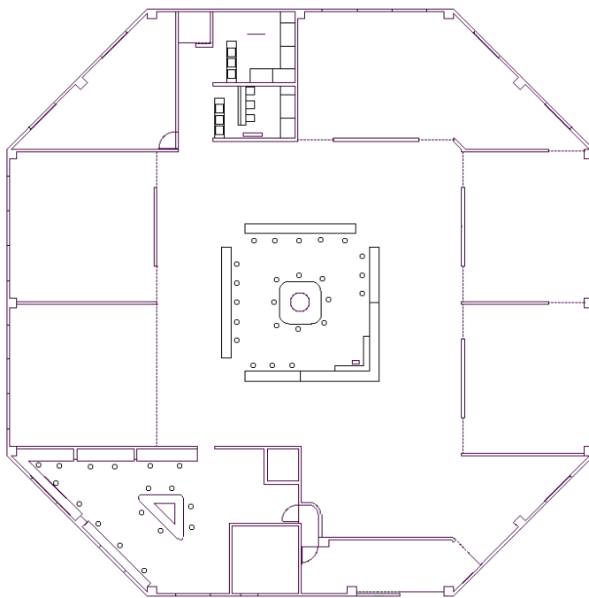
資料館 平面図
