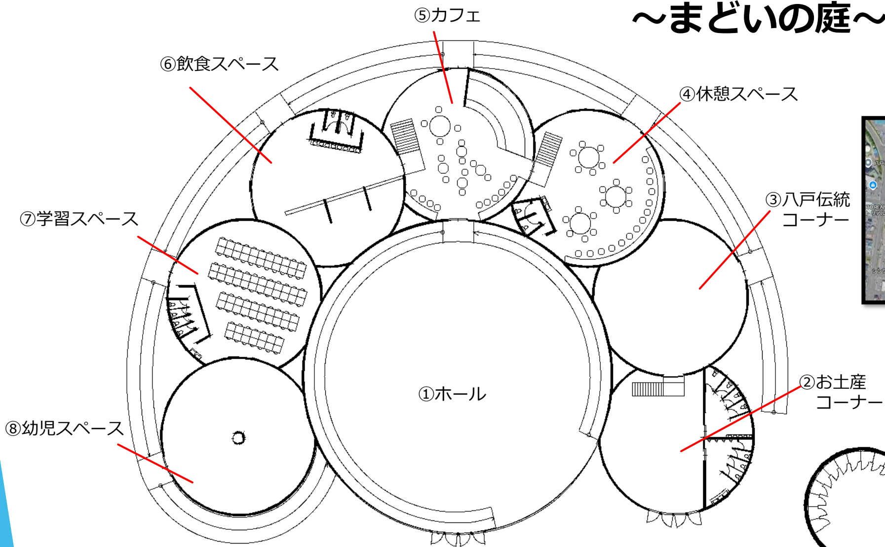
平面図
